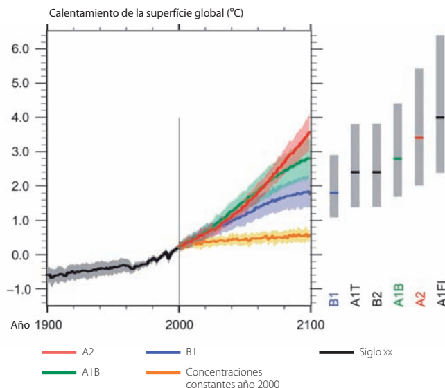
Figura SPM.5. Las líneas continuas son medias globales multimodelo del calentamiento de la superficie (en relación con el período 1980-1999) para los escenarios A2, A1B y B1, representadas como continuaciones de las simulaciones del siglo xx. El sombreado indica el intervalo de desviación estándar (+1) de las medias anuales del modelo individual. La línea naranja corresponde al experimento donde las concentraciones se han mantenido constantes a los valores del año 2000. Las barras grises de la derecha indican la mejor estimación (línea continua dentro de cada barra) y el intervalo probable evaluado para los seis escenarios de referencia del informe SRES. La evaluación del mejor valor estimado y de los intervalos probables en las barras grises incluye los AOGCM a la izquierda de la figura, así como los resultados de una clasificación jerárquica de modelos independientes y restricciones observacionales (figuras 10.4 y 10.29).
